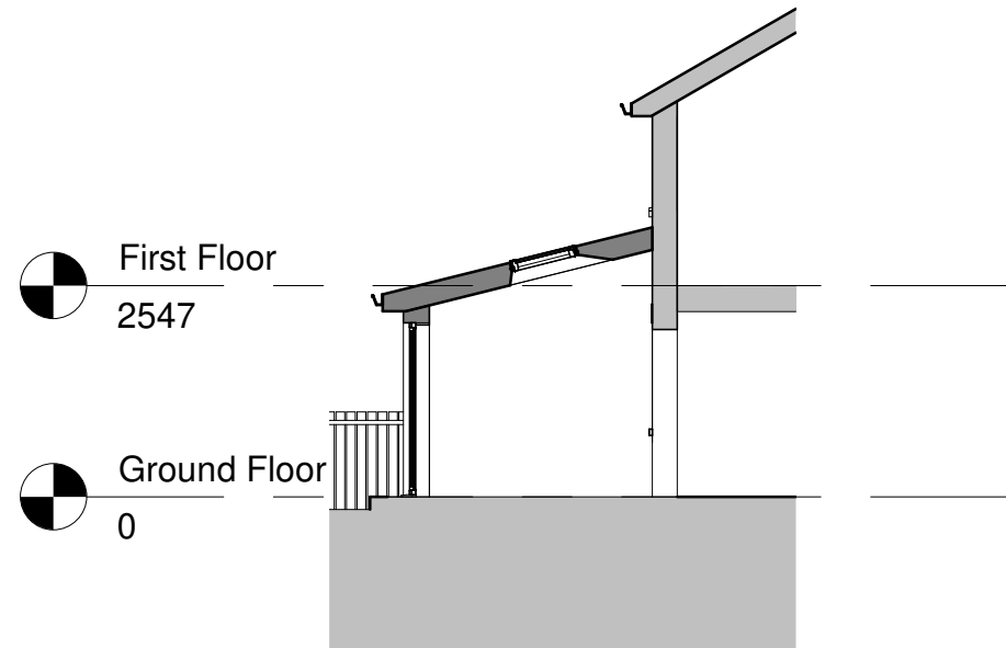
Section AA 1 : 100
